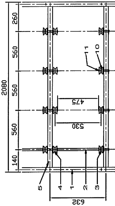
TOP ELEVATION
