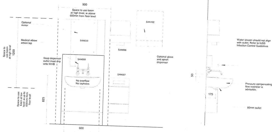
2 ELEVATION 1 : 20
