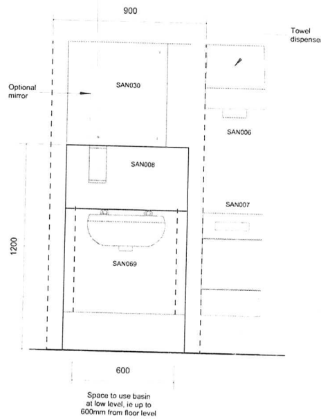
2 ELEVATION 1 : 20
