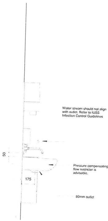
3 ELEVATION 1 : 20
